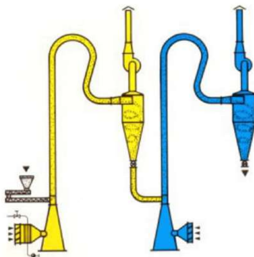
Secador e resfriador de coluna, com aquecimento a vapor, água quente ou gás. Flash dryer and cooler column with steam heating, hot water or gas.
